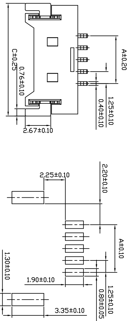
P.C.B. LAYOUT
